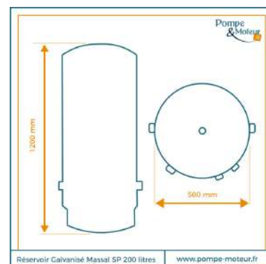
Réservoir Galvanisé Massal SP 200 litres www.pompe-moteur.fr
